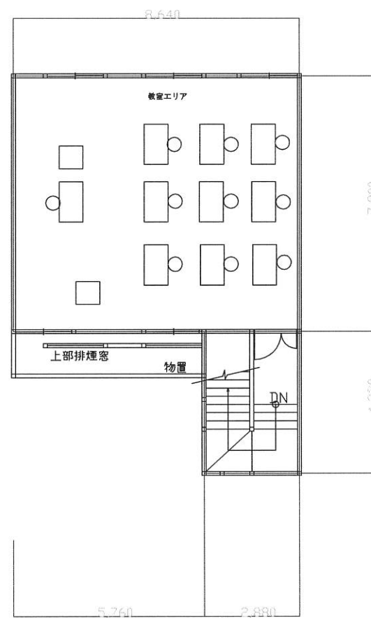
2階平面図 1/100
